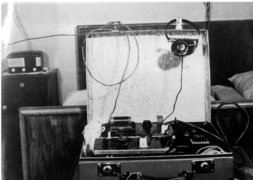
Obr. 4: Vysílačka MUDr. Josefa Zenáhlíka ve stavu, v jakém ji našla StB po Zenáhlíkově zatčení 26. dubna 1953. Jedná se o britský typ 3MK II, po válce upravený a vyráběný v západním Německu firmou Telefunken (ABS, sign. Z-10-932)
