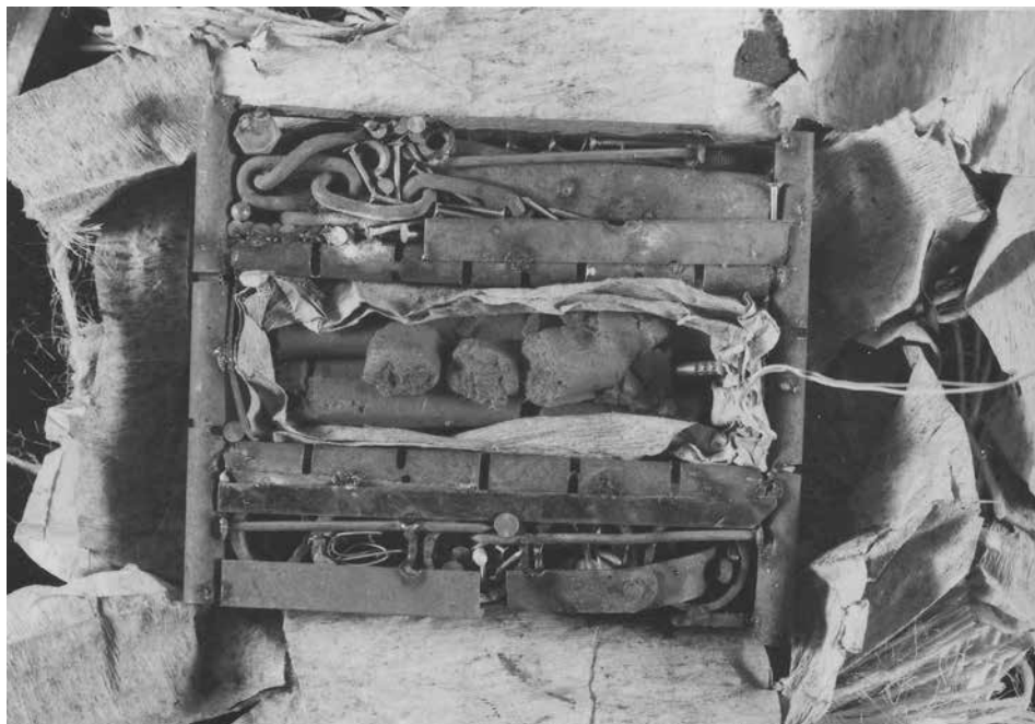
Obr. 7: Detailní pohled na rozbalené výbušné zařízení. Uprostřed je 400 g částečně rozbalené plastické trhavinu, do ní je vložena elektrická rozbuška s vodiči. Rozbuška po zapnutí elektrického proudu přivede trhavinu k výbuchu. Jiným způsobem než pomocí rozbušky nešla aktivovat. Beňo zkoušel malý kousek trhaviny v popelníku zapálit, slabě hořela a po chvíli zhasla, zbytek bez následků „uklidil“ do sporáku. Kolem plastické trhaviny je svařenec z kovového odpadu. V rámu jsou nařezané drážky, aby se při výbuchu mohl roztříštit na střepiny, vložený kovový odpad – sekané železo – ještě zvyšoval nebezpečnost nálože.
