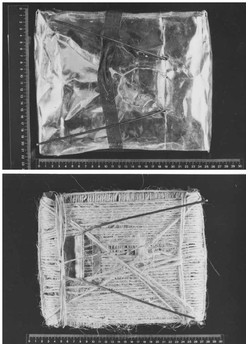
Obr. 6: Obě výbušná zařízení
