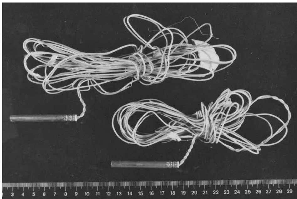
Obr. 8: Detailní pohled na rozbušky s přívodním kabelem
